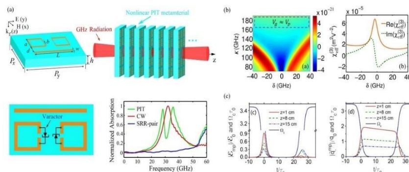
图 1 (a) 辐射场与PIT超颖原子阵列相互作用模型 (上), 和嵌入非线性元件 (变容二极管) 的超颖原子及PIT超颖原子阵列的归一化吸收谱线 (下); (b) 长波-短波的共振区域 (左), 和增强的克尔效应 (右); (c) 超颖材料中等离极化激元的有效存储和读取。
