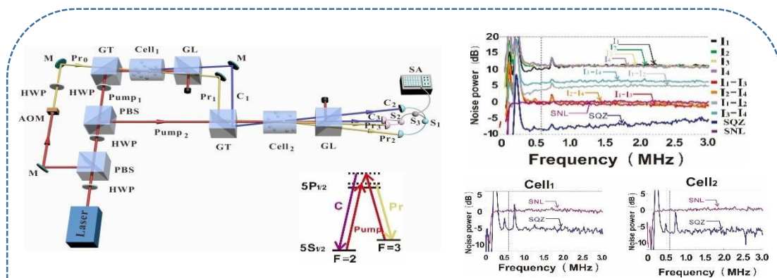
图1 利用四波混频的空间复用产生四光压缩的实验装置图及实验结果
