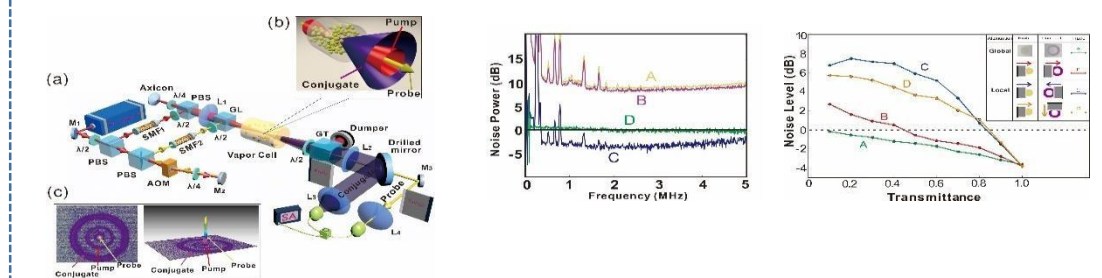
图2 利用四波混频的空间复用产生高斯模式探针光与锥形共轭光之间多模量子关联的实验装置图及实验结果
