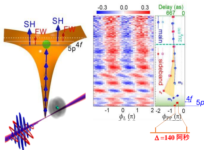
图1 原子强场多光子吸收和阿秒共振电离延时测量
