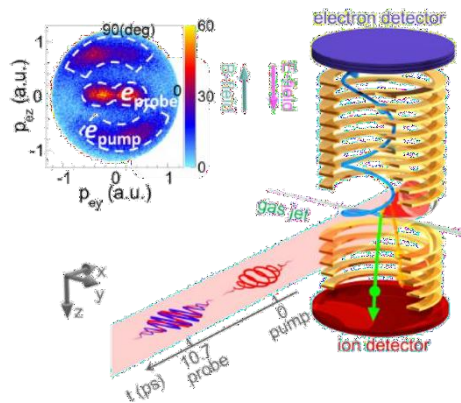
图1 泵浦-探测解耦分子电离解离过程
